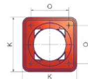
Фланец горелки
