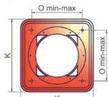
Фланец горелки
