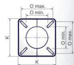
Фланец горелки
