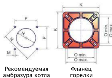
Фланец горелки
