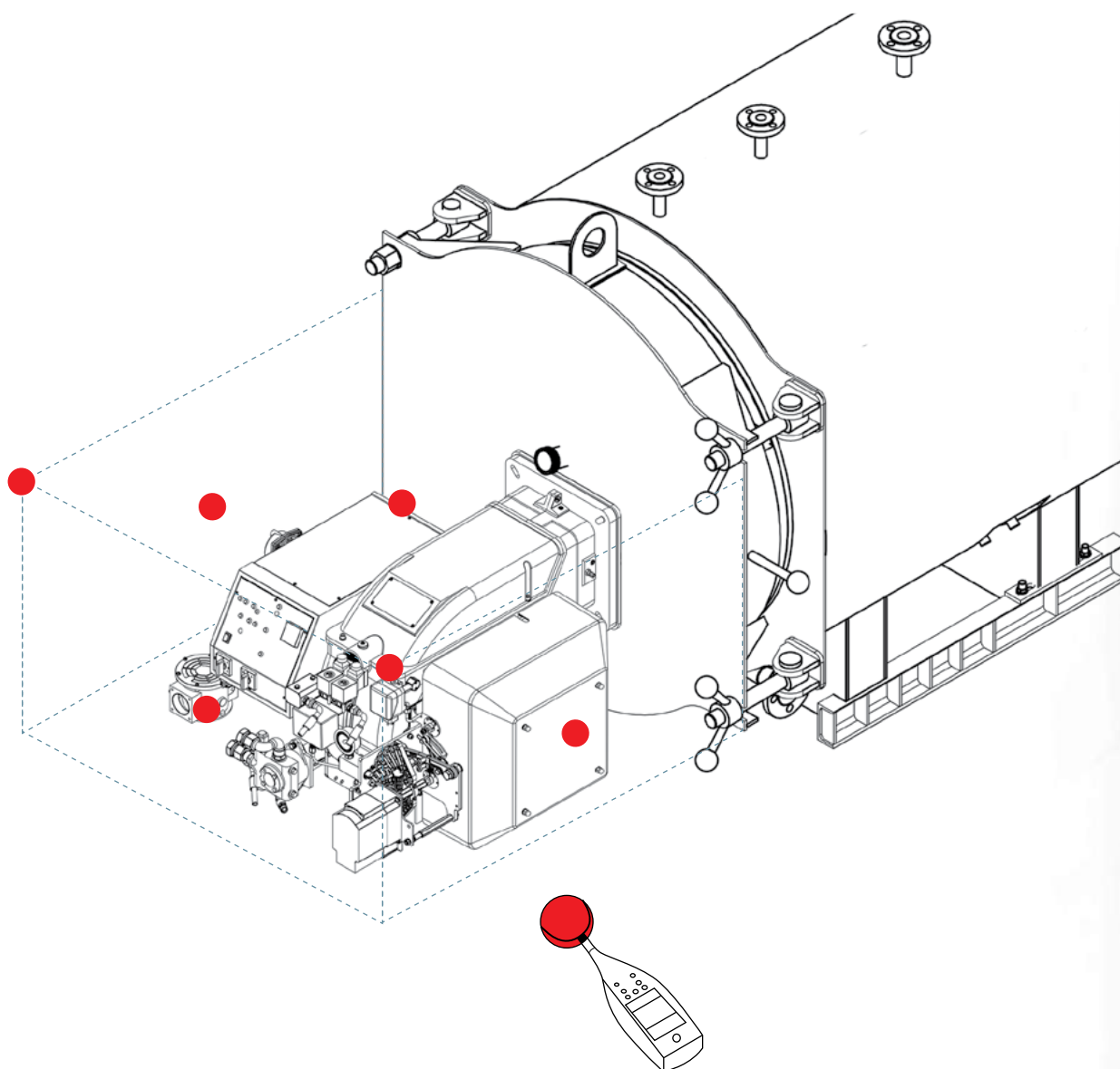
● Измерение уровня шума – расположение фонометров
